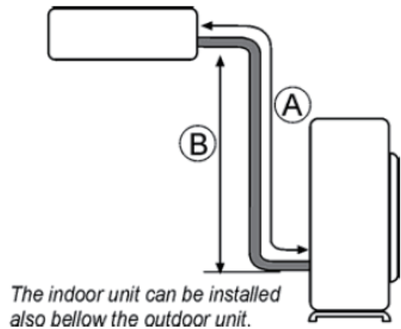
MASSIMA TUBO LUNGHEZZA E ALTEZZA (TIPO INVERTER)
