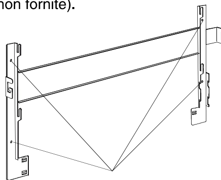
Fori di fissaggio per montaggio alla parete
