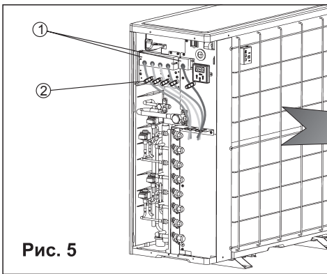
Рис. 5. 1. Разъем 2. Кабельный хомут
