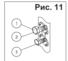
Рис. 11 1. Впускной клапан 2. Рабочий порт 3. Жидкостный клапан
