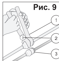
Рис. 9 1.Разводной ключ 2.Ключ с торсиомером 3.Соединение
