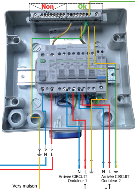
Coffret électrique AC mono <6 kWc (AirSolar) Raccordement des terres dans le coffret
