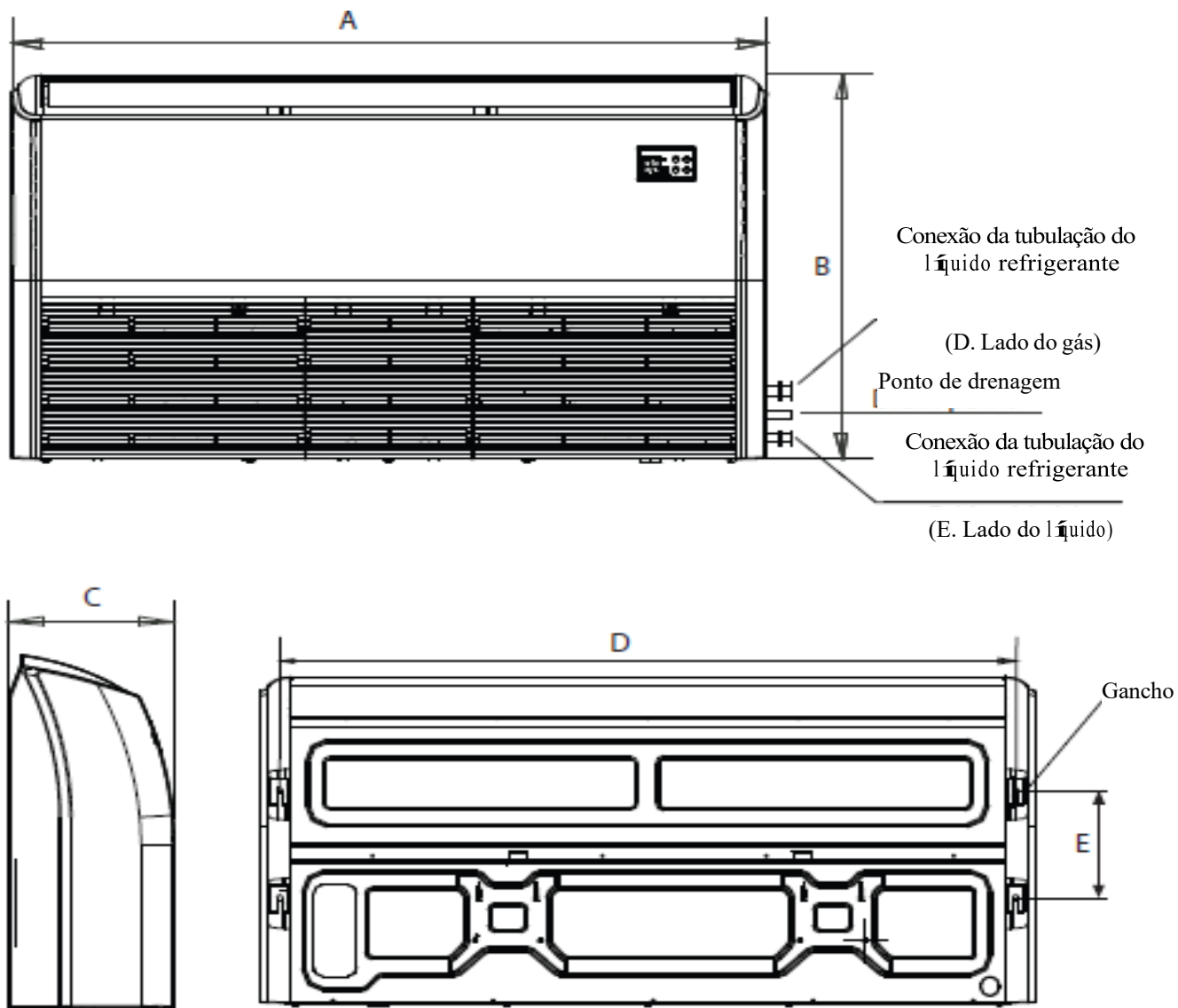
Tamanho de instalação das partes internas
