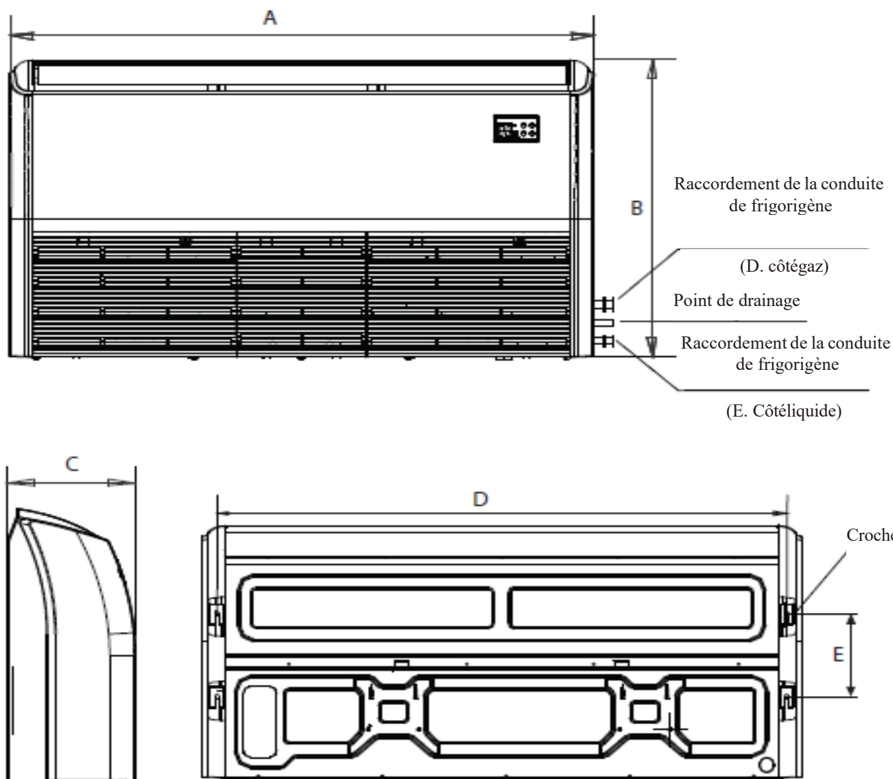
Taille de l'installation des pièces intérieures
