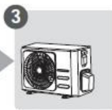
Instale la unidad externa
