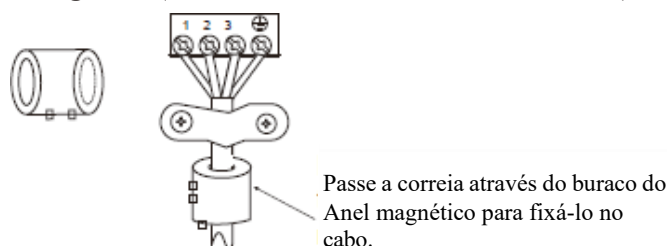
Diagrama da fiação conectiva
