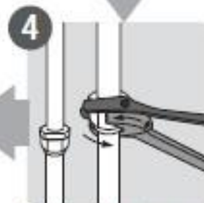
4 Raccorder les conduites de frigorigène
