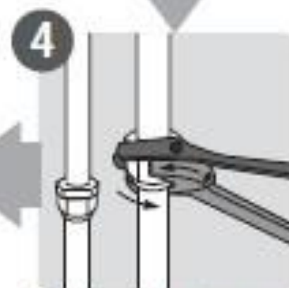
4 Verbinden Sie die Khlgasleitungen
