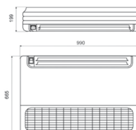
Dimensions : modèles 012-024
