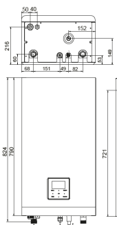
WELLEA S MT unité intérieure
