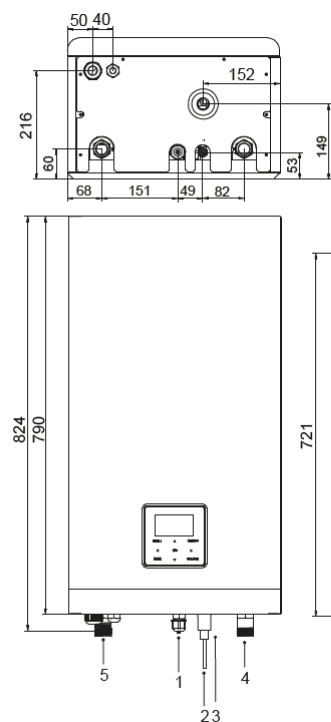
WELLEA S MT unité intérieure
