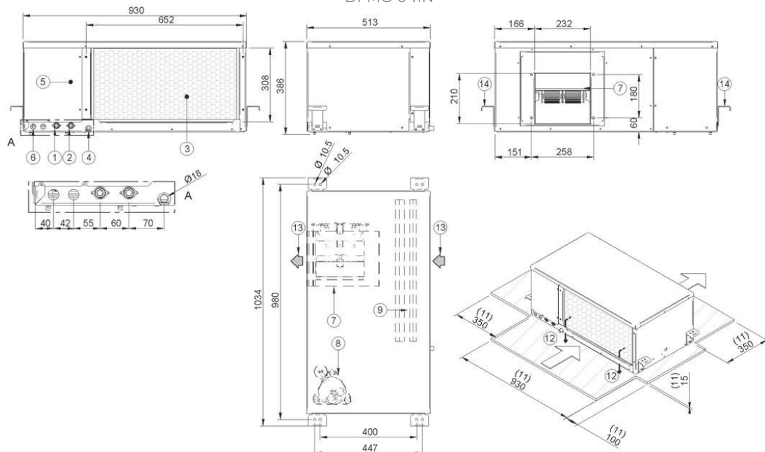
DFMO 041N
