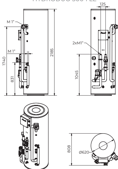
HYDRODUO 300 1 LE
