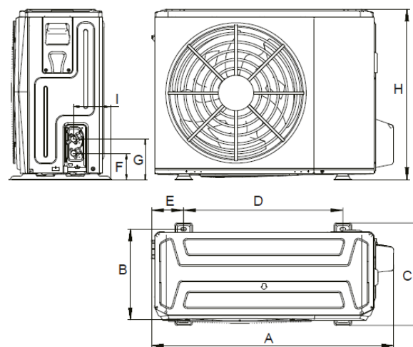
WELLEA unité ext. 4-6 kW
