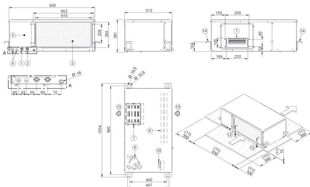
DFMO 041N
