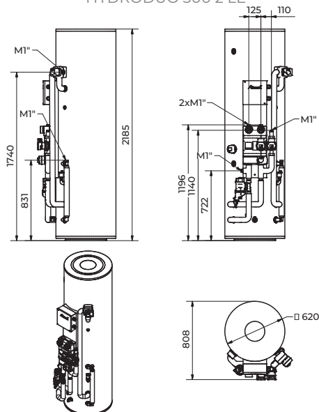
HYDRODUO 300 2 LE
