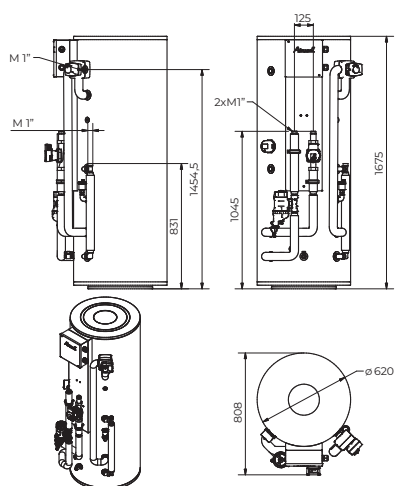
HYDRODUO 300 1 LE
