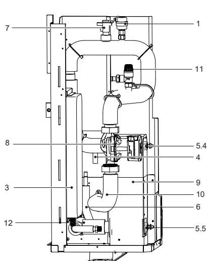
8~16 kW con riscaldatore di backup
