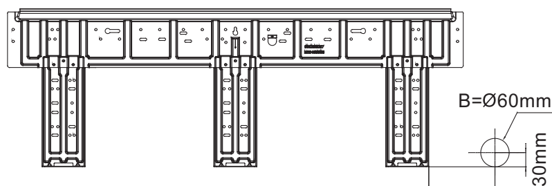
HVVA-070/090N-01M22
