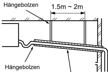
Gefälle von 1/100 oder mehr
