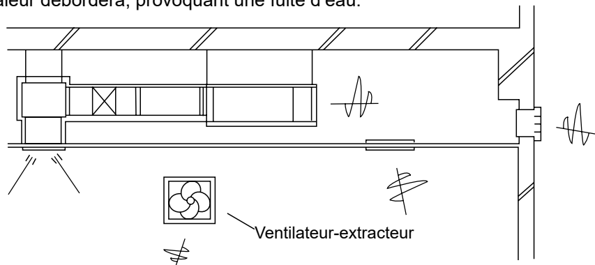
Exemple de mauvaise installation
