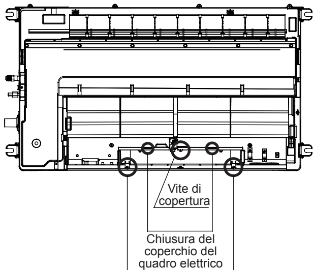
Le due viti per la scatola di fissaggio
