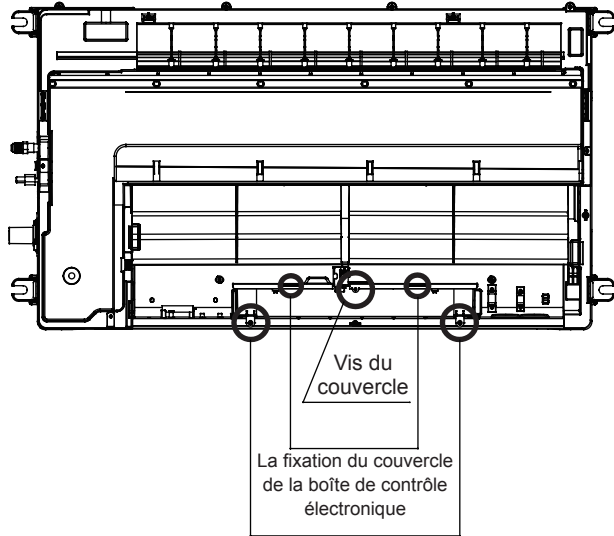
Deux vis pour la fixation de la boîte
