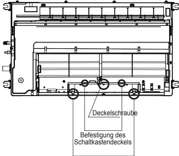
Zwei Schrauben zur Befestigung des Kastens
