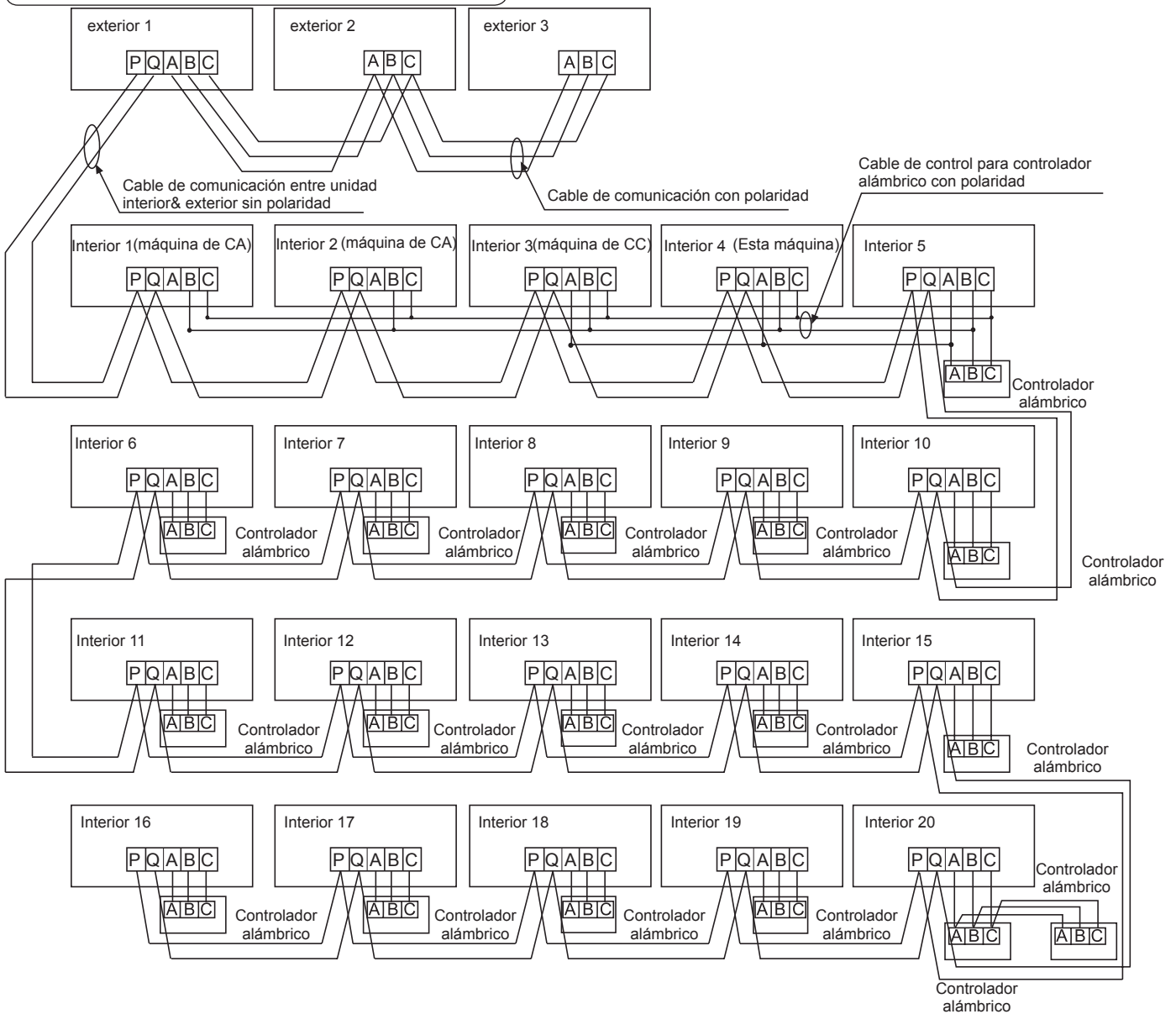
Diagrama de Cableado del Cable de Señal
