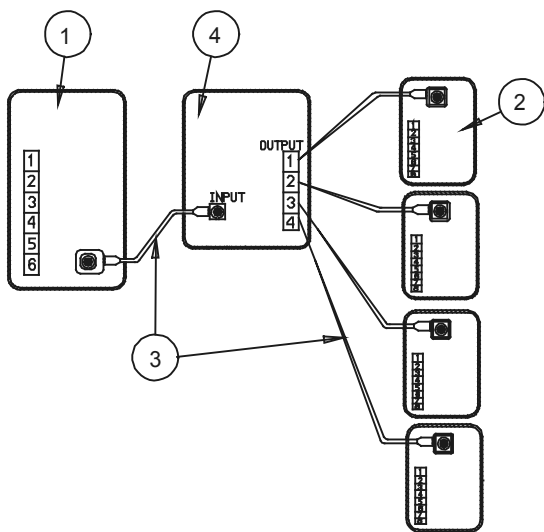
Figura 19: Collegamento di 4 pannelli di controllo visivo in parallelo (opzionale)
