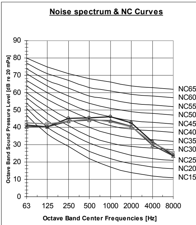
ELSI-RSF045-N13 Cooling
