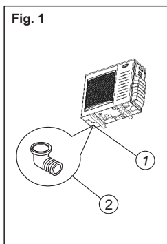
Fig. 1 1. Dessous de l'unité extérieure 2. Raccord d'évacuation des condensats
