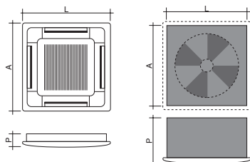
U.I.: AE EKF 24 / EKF 30-45 T
