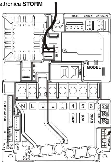
Scheda elettronica STORM
