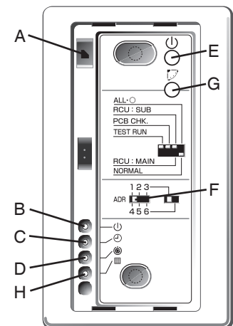
Extern installierte Signalempfänger ST-NDLP/-NDHP/-NF(M)FL
