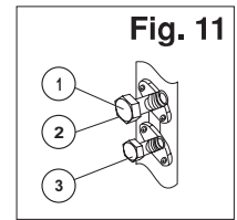
Fig. 11 1. Válvula de aspiración. 2. Tapón de servicio. 3. Válvula de líquido
