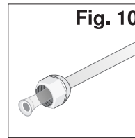
Fig. 10 Para prevenir la salida de refrigerante, cubra la superficie señalada con aceite de refrigerante.
