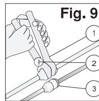
Fig. 9 1. Llave 2. Llave fija 3. Unión
