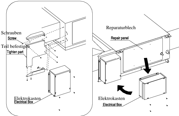
Schaltbild für die Teile des Elektrokasten
