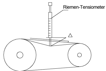
Abb. 26 Nutzung des Riemen-Tensiometers
