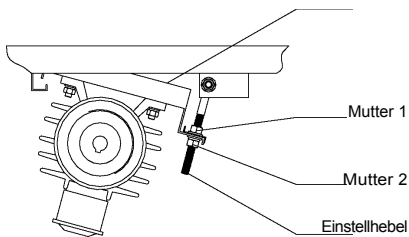
Abb. 25 Einstellung der Spannkraft des Riemens
