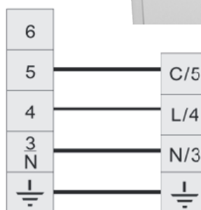
Unité extérieure
