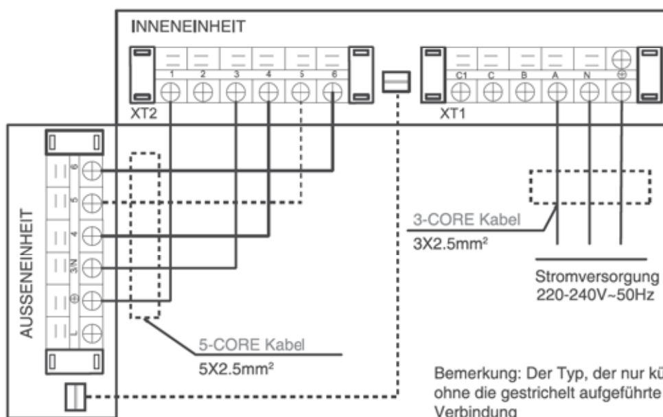
Zeichnung 36: Stromversorgung des Innengeräts
