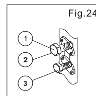
Fig. 24 1. Válvula de succión 2. Abertura de servicio 3. Válvula de líquido
