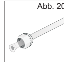
Abb. 20 Bestreichen Sie die Bördelflächen mit Kältemaschinenöl, um ein Kältemittelleck zu vermeiden.
