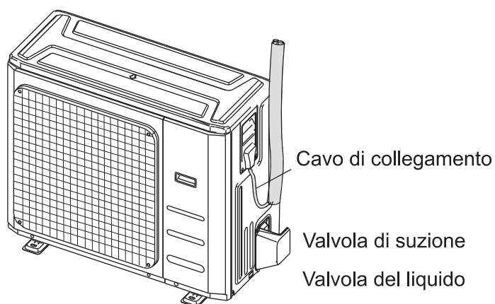
Unità esterna
