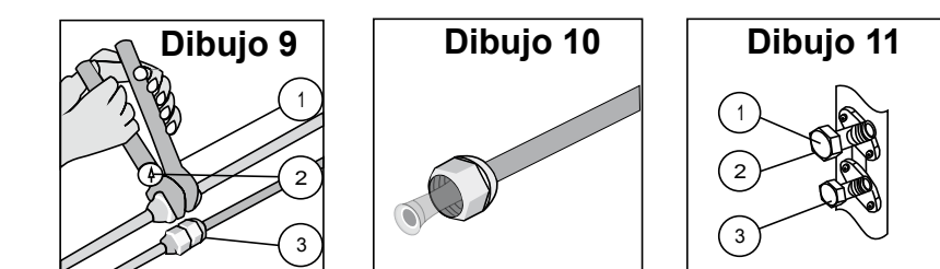
Dibujo 9 1. Llave 2. Llave fija 3. Unión Dibujo 10 Para provenir la salida de refrigerante, cubra la superficie señalada con aceite de refrigerante. Dibujo 11 1. Válvula de aspiración. 2. Tapón de servicio. 3. Válvula de líquido
