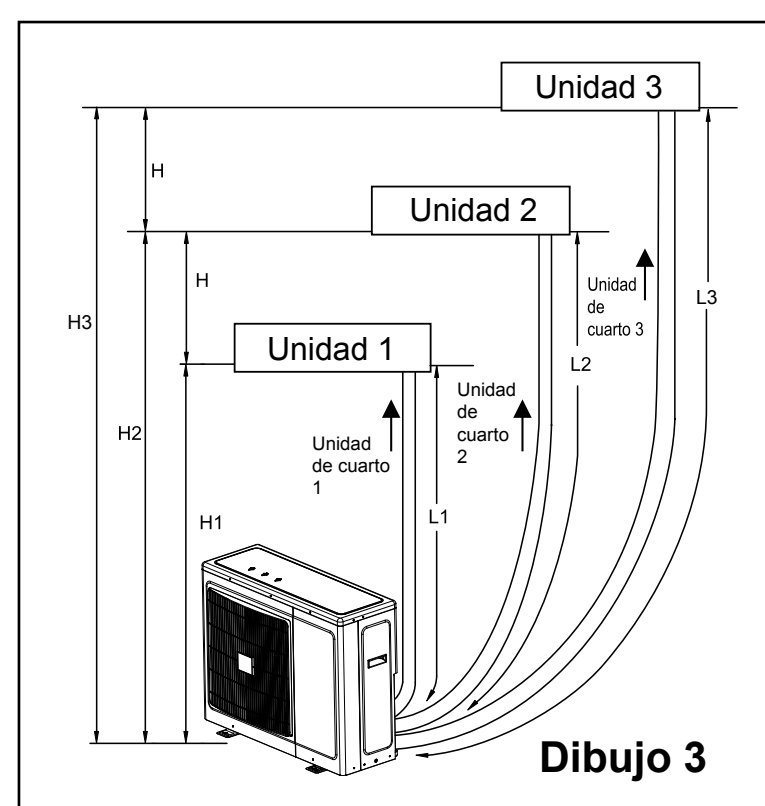
Dibujo 3 Observaciones: L1+L2+L3 ≤ 35m y L1, L2, L3 ≤ 25m H ≤ 5m H1, H2, H3 ≤ 15m No es necesario tener una carga adicional.
