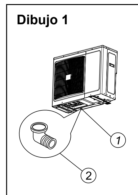
Dibujo 1 1. Fondo de la unidad exterior 2. Codo de drenaje.
