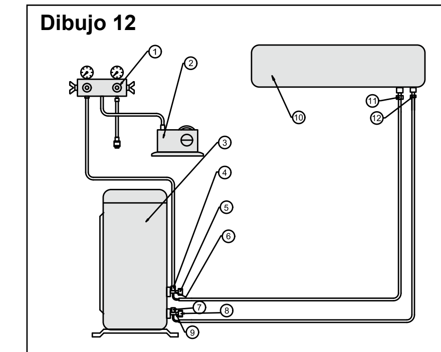
Dibujo 12 Puente de manómetros Bomba de vacío UNIDAD EXTERIOR Obús Casquillo Válvula de aspiración Obús Tapón Válvula de líquido UNIDAD INTERIOR Conexión de llamada de succión Conexión líquida de * En algunos modelos solamente
