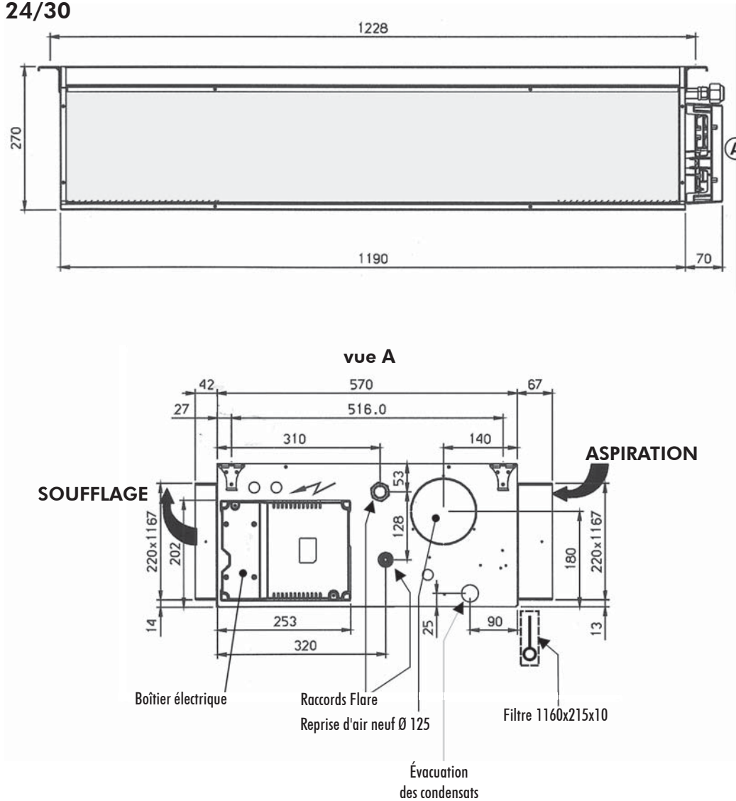
Caisson de traitement BS 24/30
