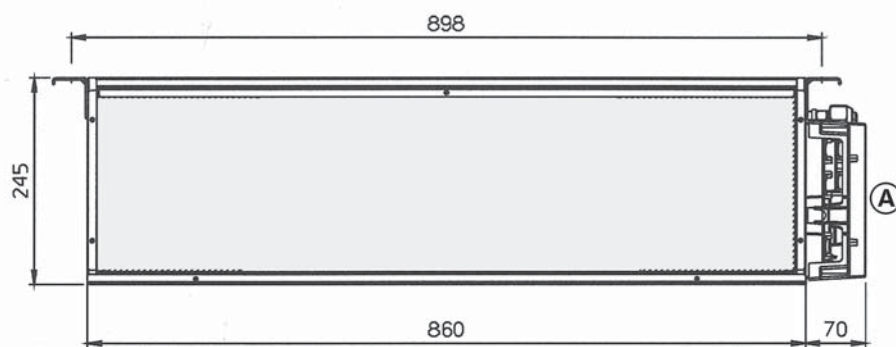
Caisson de traitement BS 11/15/18
