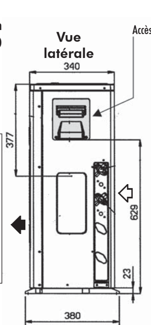
Groupe de condensation GCN 30
