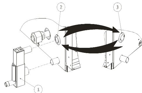
Figura 6: Sifone sulla linea di drenaggio (optional)
