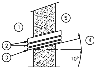
Figura 8: Cavo e tubi di connessione
