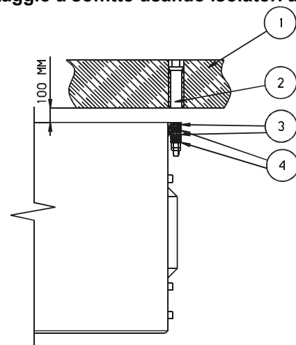
Figura 4: Installazione dell'unità interna Montaggio a soffitto usando isolatori a molla
