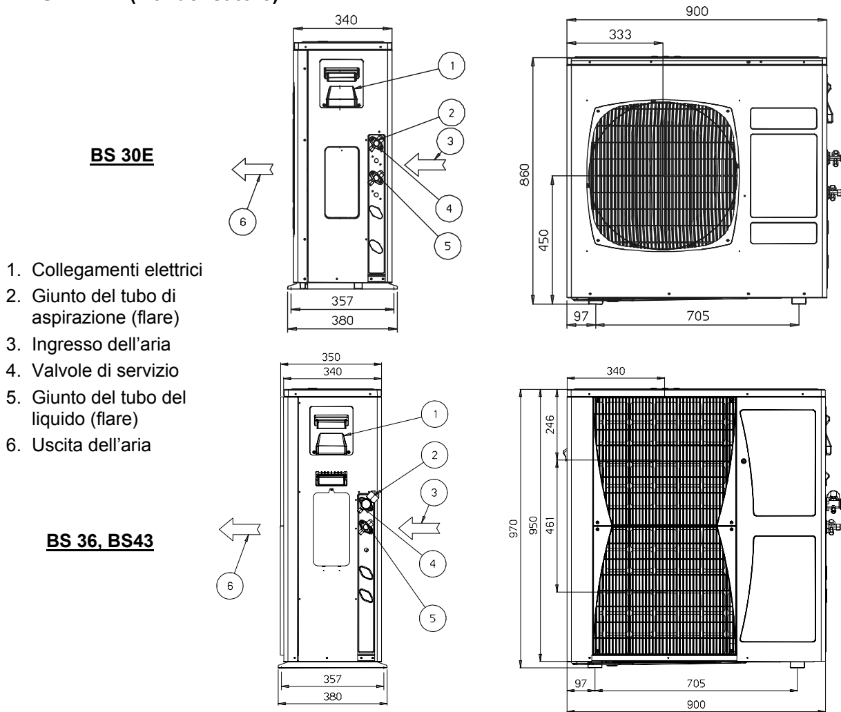
Figura 2: Modelli BS - Dimensioni Generali
