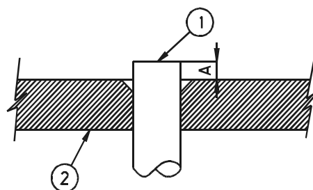
Figura 14: Svasatura del tubo
